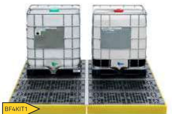
BF4KIT1B o BF4KIT1Y - 4 x BF4B (BF4Y), 2 x BFS2, 2 x BFS4 & 4 x BFC
